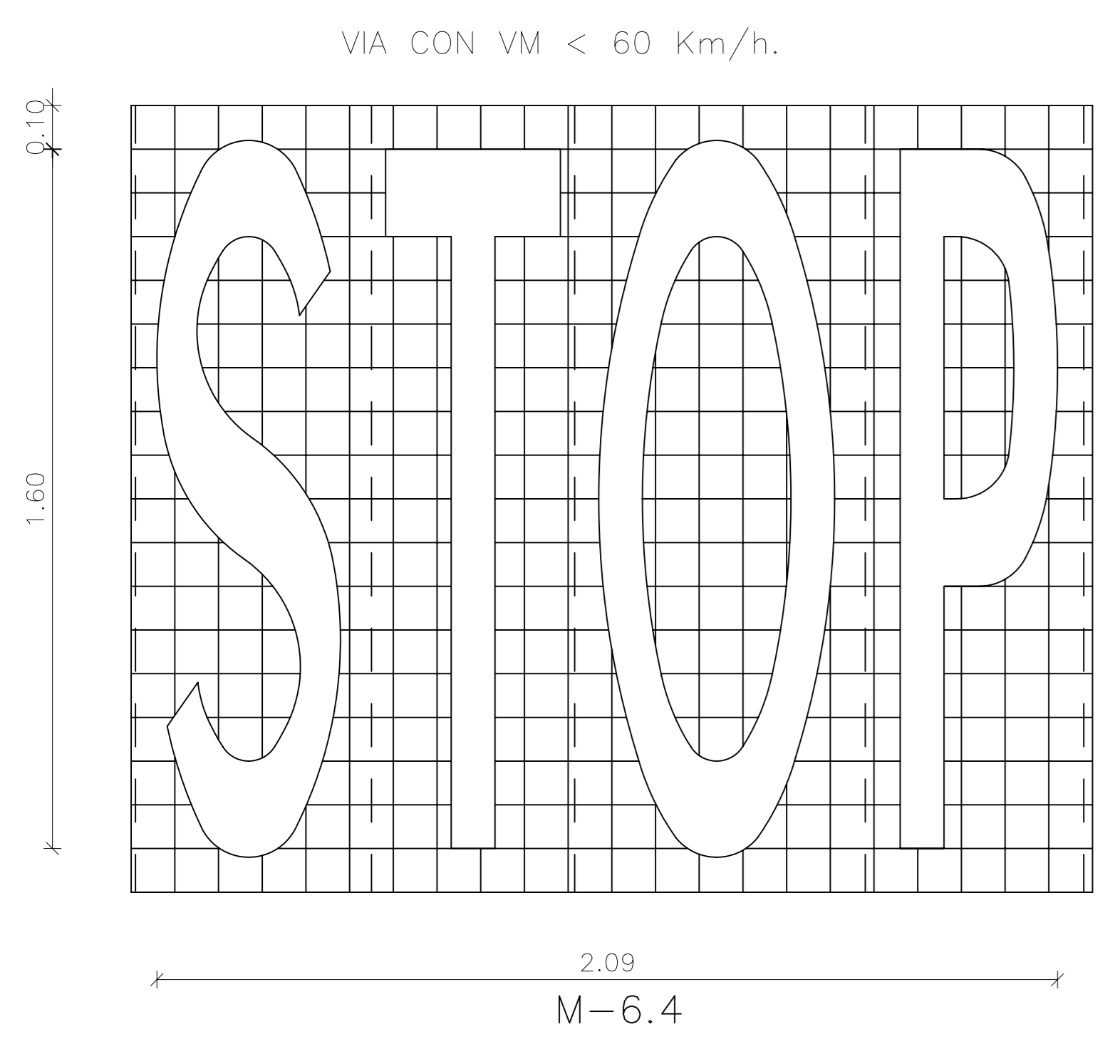
LEYENDA MARCAS VIALES NORMA 8.2. I.C. E 1:125
